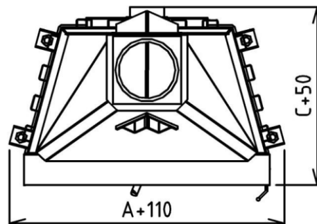
Krb. vložka standard - přední sklo
