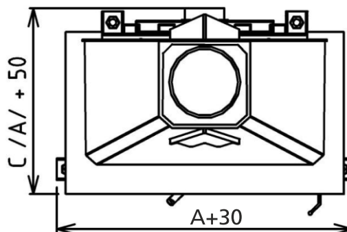
Krb. vložka třístranná
